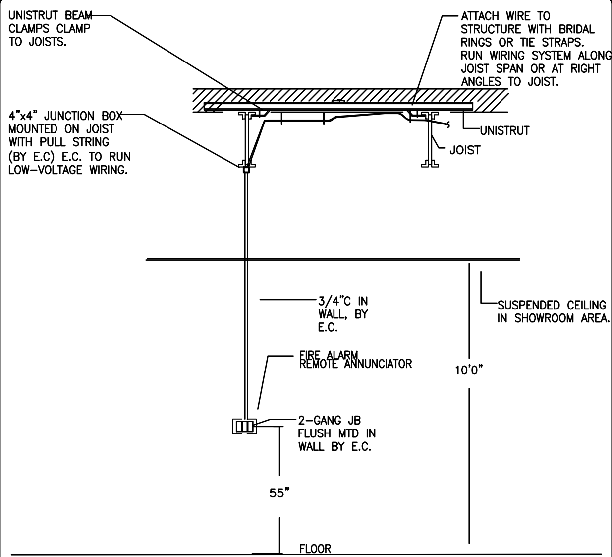
8 REMOTE ANNUNCIATOR MOUNTING N.T.S.
