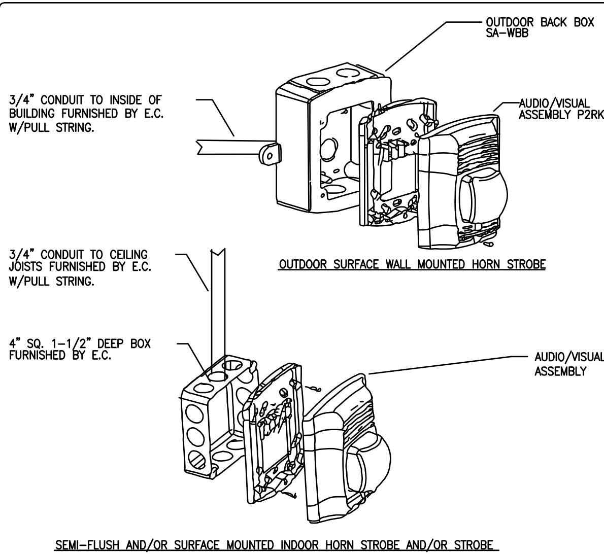
1 FIRE ALARM AUDIO/VISUAL DETAIL N.T.S.
