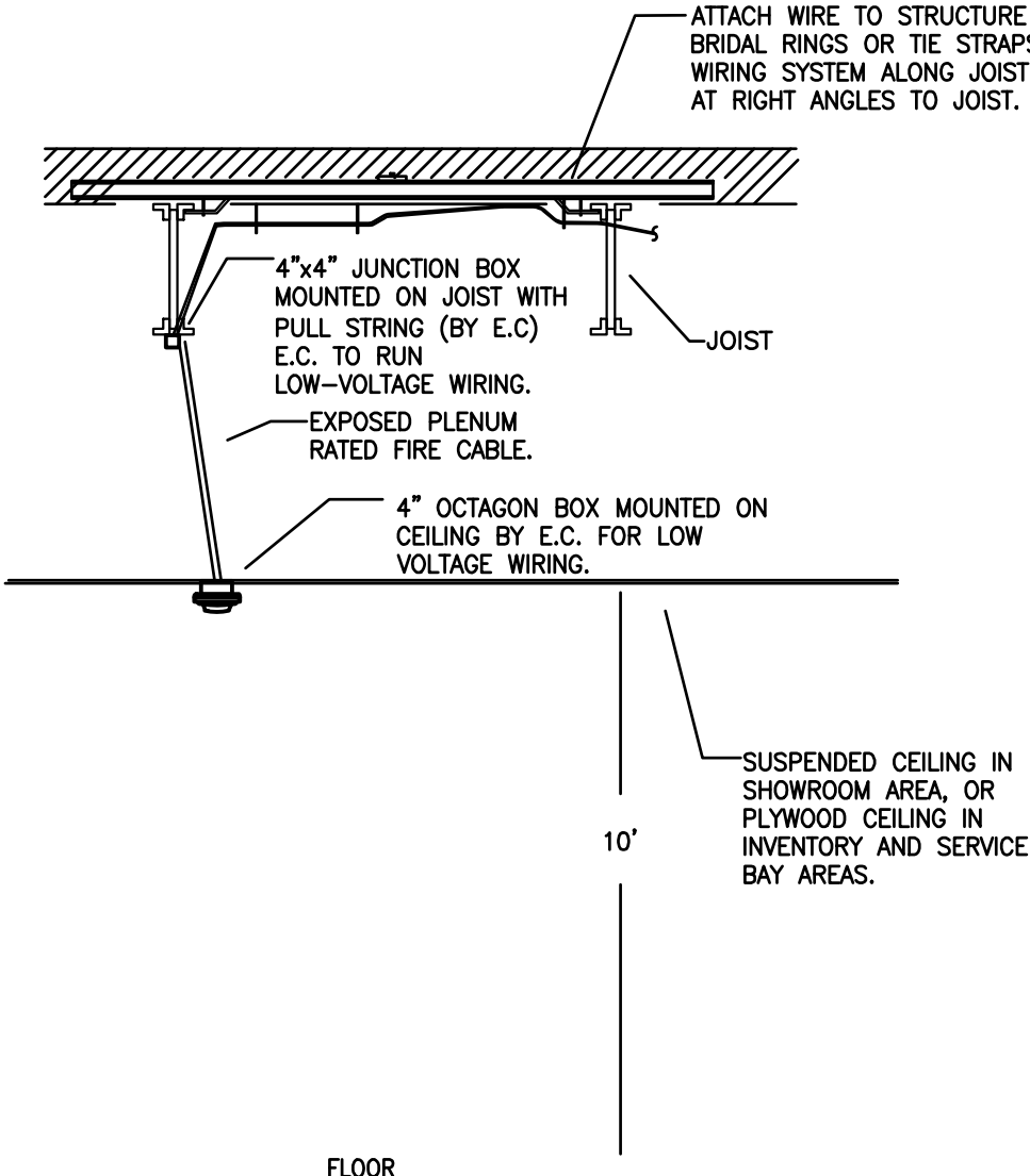
3 SMOKE DETECTOR MOUNTING N.T.S.
