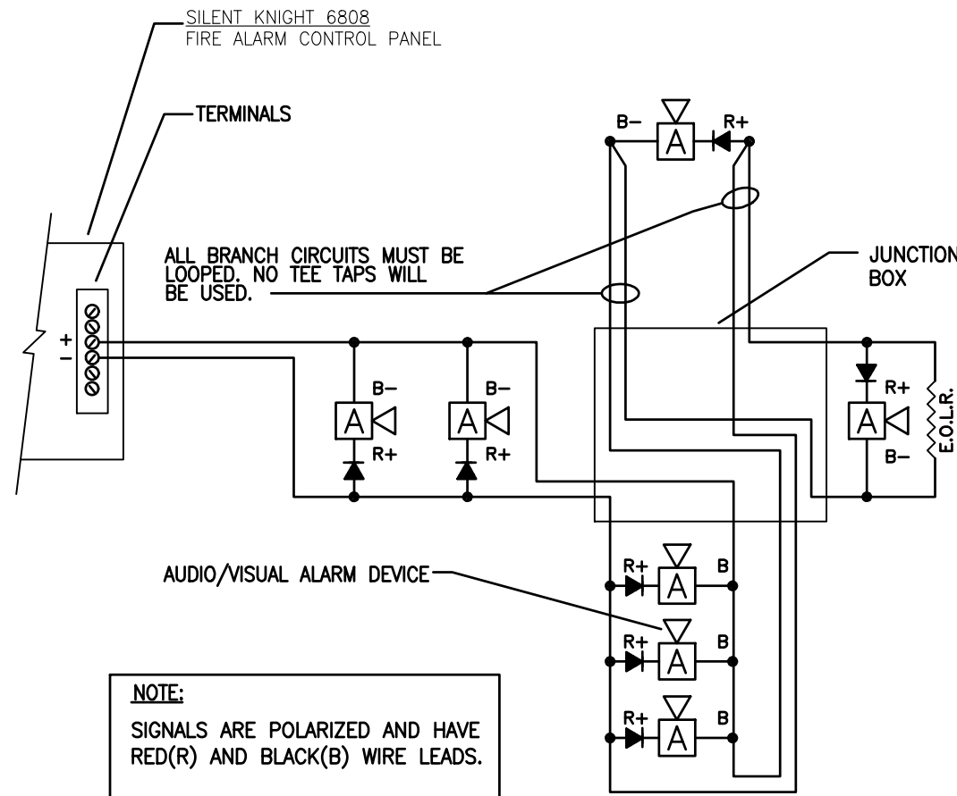
1 FIRE ALARM AUDIO/VISUAL DETAIL N.T.S.
