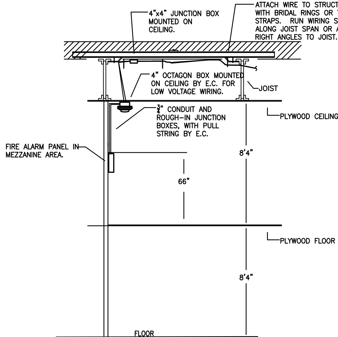
6 FIRE PANEL MOUNTING N.T.S.
